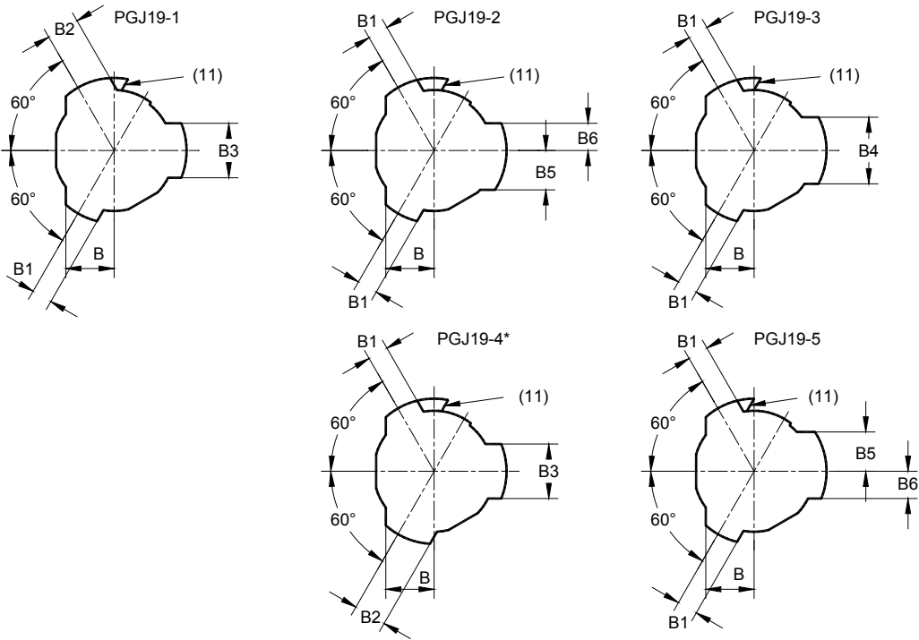
Connectors Connecteurs PGJ19-1, PGJ19-2 & PGJ19-3
